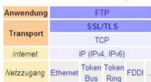
FTPS im TCP/IP-Protokollstapel:
